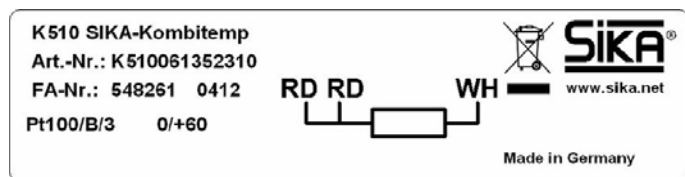
Beispiel Typenschild
