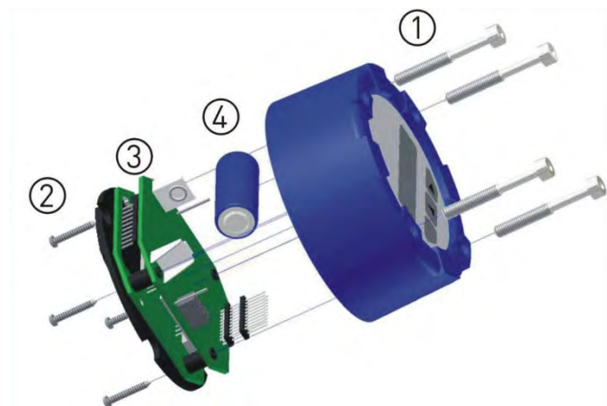
Explosionszeichnung Anzeigeeinheit 1
