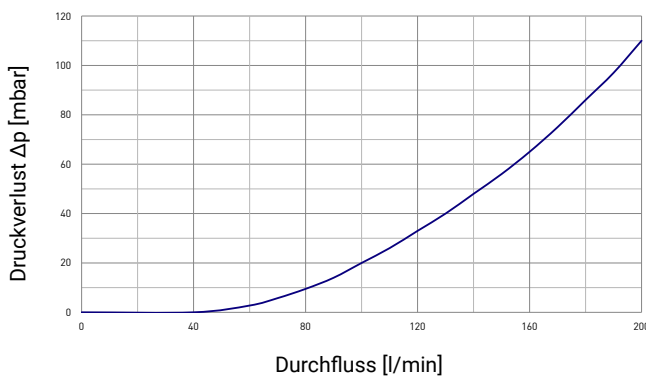
Typischer Druckverlust VMZ20
