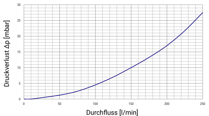
Typischer Druckverlust VMZ25
