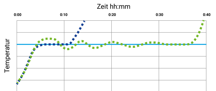
Ohne Raketenregler: Lange Einschwingzeit auf die Zieltemperatur Mit Raketenregler: Einschwingzeit auf Zieltemperatur um ca. 90% reduziert
