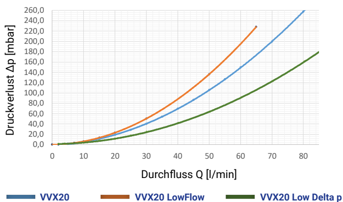
Typischer Druckverlust VVX20
