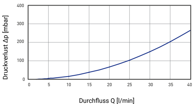
Typischer Druckverlust VVX15
